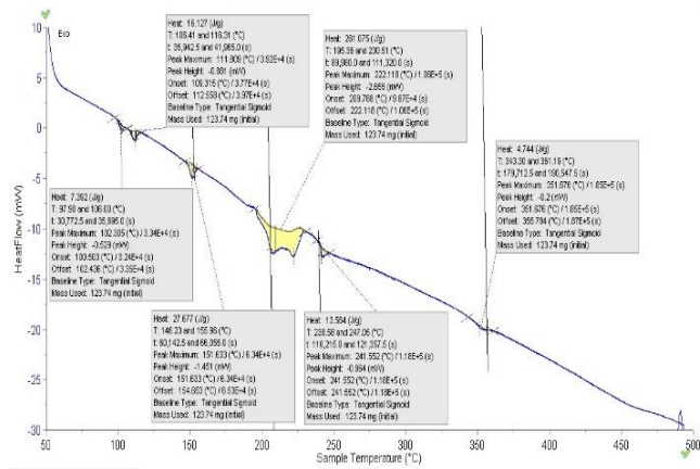
Расми 1. Қачхаттаҳои ҳароратии намунаҳои кони «Тоҷикистони Марказӣ»
